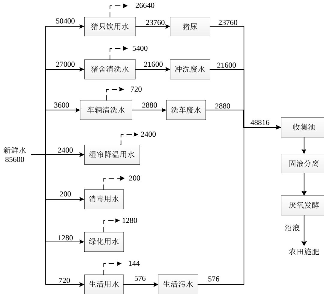
图 3.3-4 项目水平衡图(单位: \text{m}^3/\text{a} )
