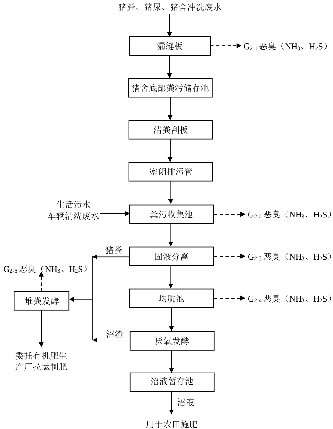
图 3.3-2 粪污处理工程工艺流程图
