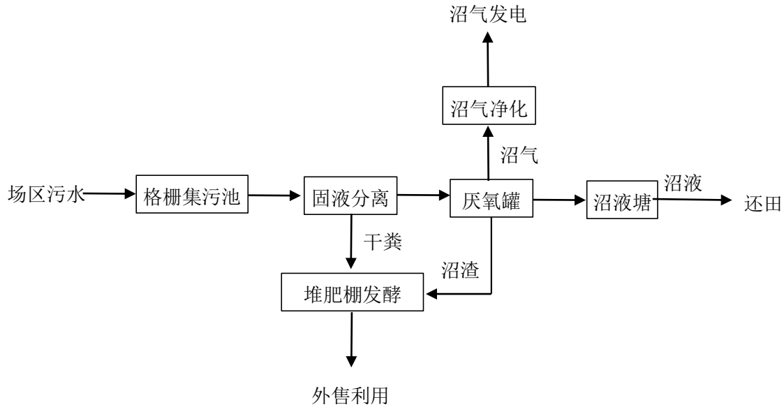
图 6.2-1 本项目污水处理工艺流程图
